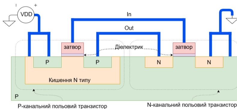
Рис. 1. КМОН інвертор на підкладці р-типу
